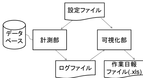
図 1. TaskPit のシステム構成
